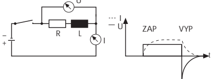
Obr. 2 Průběh proudu a napětí při zapínání cívky relé
