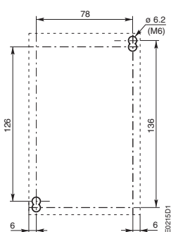
AE 95, AE 110, TAE 95, TAE 110 - plán vrtání otvorů
