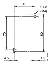
AL 30, AL 40, TAL 30, TAL 40 plán vrtání otvorů
