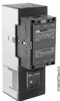
Stykač A185 s relé E 200 DU a krytem svorkovnice LT 200 E
