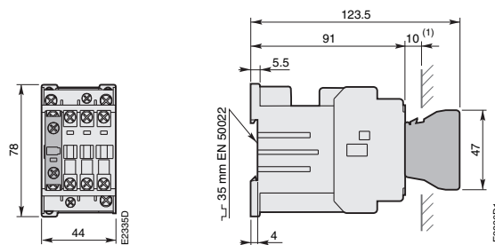
AL 9 ... AL 16, AL...Z.. TAL 9 ... TAL 16 + 1-pólový blok pomocných kontaktů pro čelní montáž CA-5
