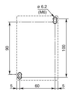
plán vrtání otvorů
