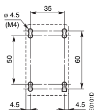
UA 16 plán vrtání otvorů
