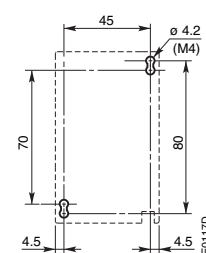
plán vrtání otvorů
