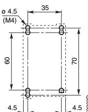
AL 9 ... AL 16 TAL 9 ... TAL 16 + 4-pólový blok pomocných kontaktů pro čelní montáž CA-5
