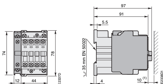
AL 9 ... AL 16 TAL 9 ... TAL 16 + 2-pólový blok pomocných kontaktů pro boční montáž CAL-5
