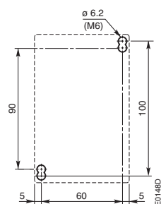
AE 50, AE 63, AE 75, TAE 50, TAE 75 - plán vrtání otvorů
