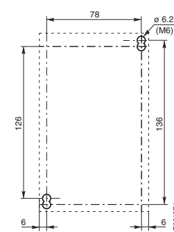
plán vrtání otvorů
