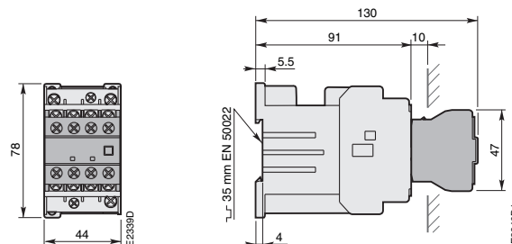
AL 9 ... AL 16 TAL 9 ... TAL 16 + 4-pólový blok pomocných kontaktů pro čelní montáž CA-5
