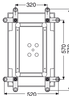
konzola
