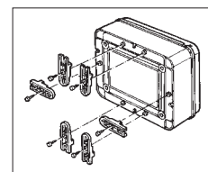
Snadná instalace izolačního kompletu použitím úchytů GW 44 621 nebo krytek na šrouby GW 44 622 / GW 44 623.
