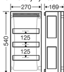
rozměrový výkres
