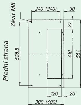
ON-2I.../300 (400) nahoře i dole
