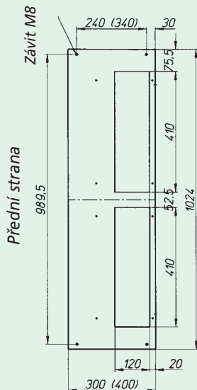
ON-5I.../300 (400) nahoře i dole
