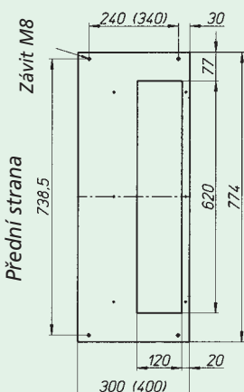
ON-3I.../300 (400) nahoře i dole
