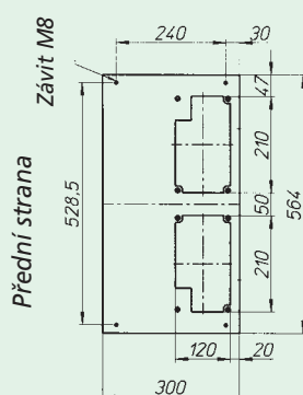
OFN-2I.../300 nahoře i dole
