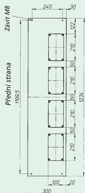
OFN-5I.../300 nahoře i dole
