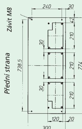
OFN-3I.../300 nahoře i dole
