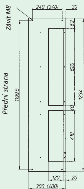
ON-5I.../300 (400) nahoře i dole
