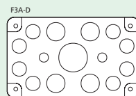
F3A-D Vložka příruby z pěnové pryže, 40 kabelů o průměru 10-13 mm, 4 kabely o průměru 17-21 mm, 2 kabely o průměru 27-30 mm
