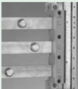
Snadná montáž přípojníc SS-30X5/60 - vhodné řešení pro montáž přípojnicového adaptéru SAD
