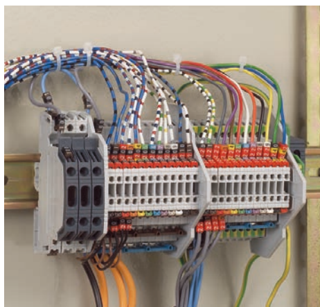
► Uspořádání kabelových svazků pomocí vyvazovacích pásek.
